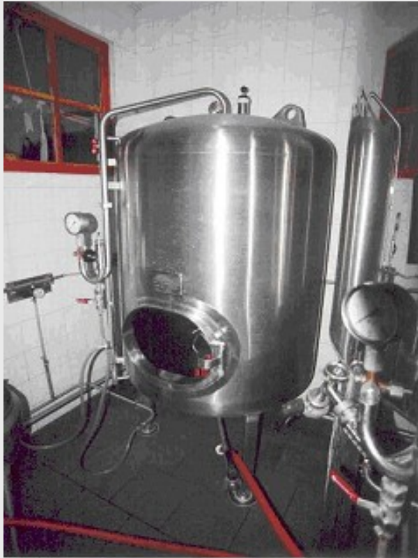
Напорный танк
