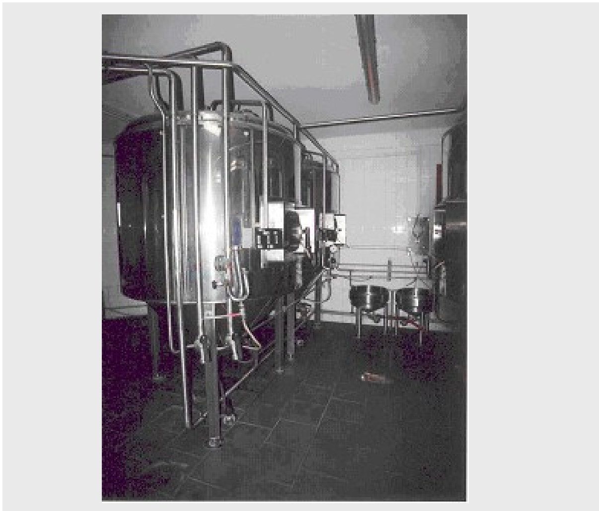
ZKTs y tina de levadura
