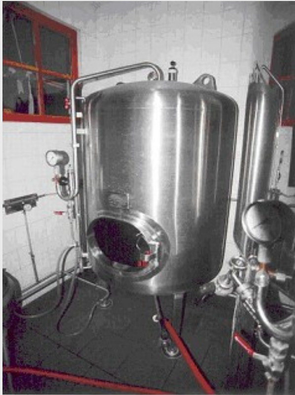
Tanque de gobierno
